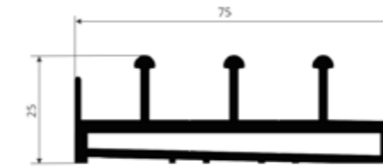
CARRIL INFERIOR SOBRE SUELO Above ground Bottom track
